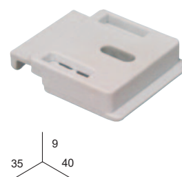
SUPPORT PLAFOND AUTOMATIQUE
