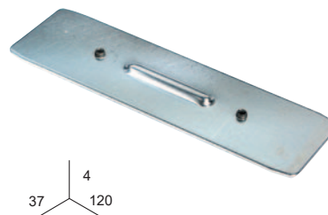
JONCTION PROFILÉS 4 ET 5 VOIES
