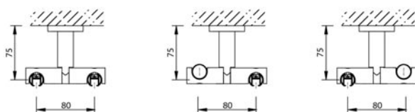
SUPPORT PLAFOND DOUBLE AUTOMATIQUE PIVOTABLE 4496
