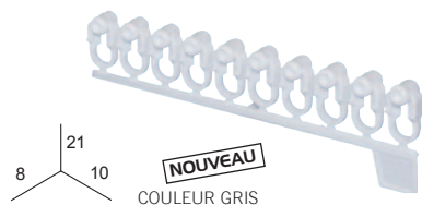
SUSPENDEDUR À ROUE. BLANC ET GRIS
