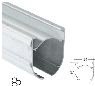
PROFILÉ 7347
