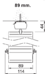
COMMANDE DROITE OUVERTURE à GAUCHE
