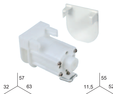
COMMANDE 1:4 + EMBOUT
