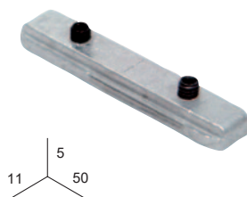
JONCTION METALLIQUE (profilés 950/910)
