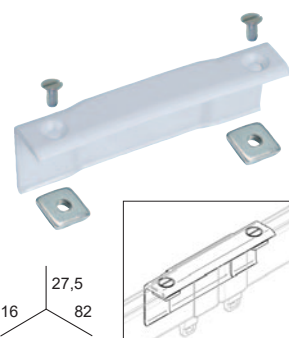
JONCTION GARNITURE POULIE
