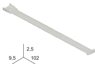
TIGE D'ÉCARTEMENT 9 cm.
