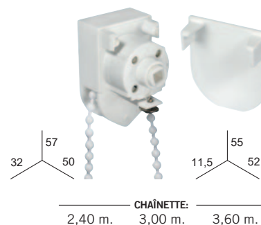
COMMANDE À CHAÎNETTE 1:2 + EMBOUT
