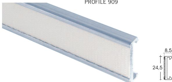
PROFILÉ 909
