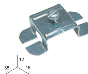
ETRIER POUR EQUERRES (Pour refs. 7187060 et 7188060)
