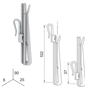
AGRAFE RÉGLABLE LONGUE
