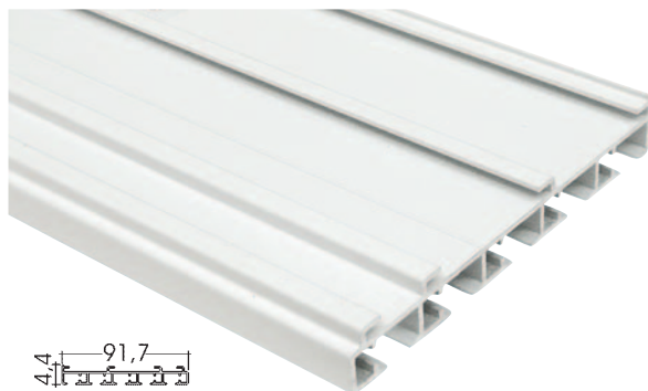
PROFILÉ 5 VOIES DE 4 m.
