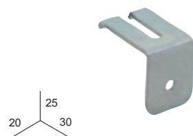
EQUERRES
