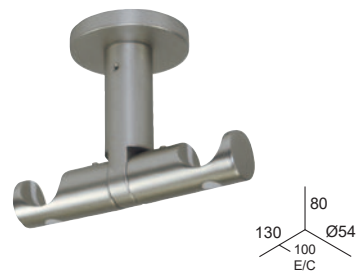
SUPPORT PLAFOND DOUBLE 20-20 mm. (Seulement disponible en nickel mat, blanc et noir)
