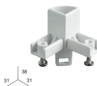
UNION D'ANGLE
