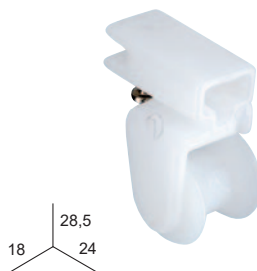
GUIDE FIL À ROUE (Pour profilés 7393 et 864)
