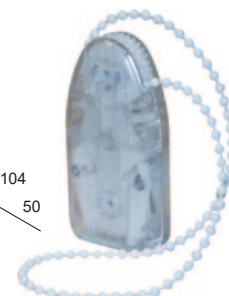
DISPOSITIF CHÂÎNETTE À DÉCLIPSAGE RAPIDE
