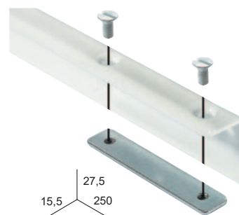
JONCTION PROFILÉ
