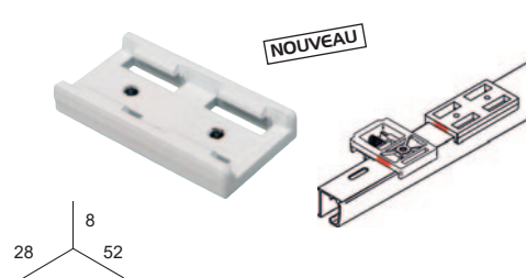
JONCTION (À utiliser avec SUPPORTS PLAFOND)
