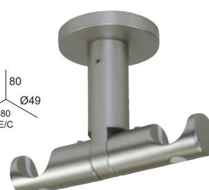
SUPPORT PLAFOND DOUBLE 20-20 mm. (Non disponible en blanc, noir, doré et doré mat)
