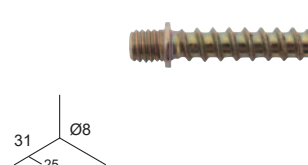
PATTE A VIS POUR SUPPORT Ø50
