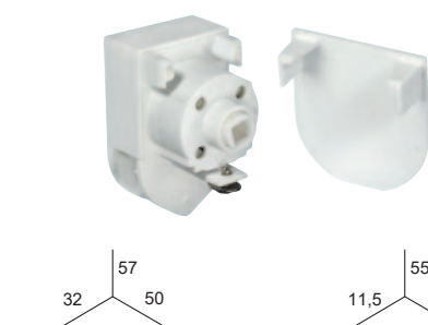
COMMANDE 1:2 + EMBOUT
