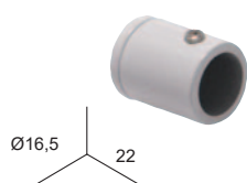
SUPPORT NAISSANCE
