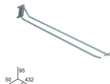
BROCHE AVEC PORTE-ÉTIQUETTE "F"
