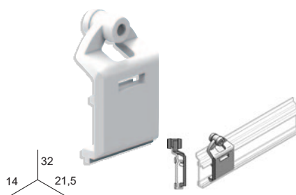
SUSPENDEUR
