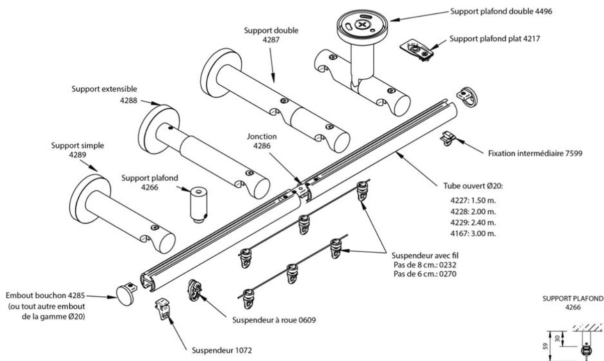
SUPPORT EXTENSIBLE AUTOMATIQUE 4288
