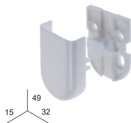
POULIE DE SÉCURITÉ RÉGLABLE POUR CHÂINETTE. BLANC
