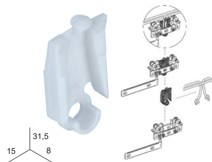
BRIDE POUR CORDON
