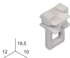
SUSPENDEDUR SIMPLE (à jumeler avec la tige d'écartement)
