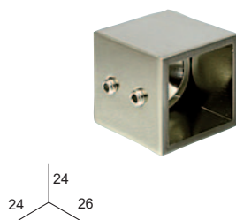
SUPPORT NAISSANCE
