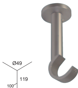
SUPPORT MIXTE MUR-PLAFOND (Non disponible en doré et doré mat)
