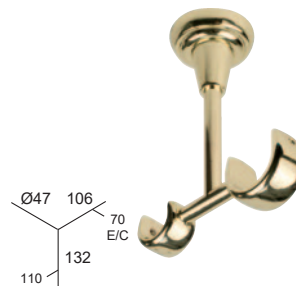
SUPPORT PLAFOND DOUBLE 28-20 mm. (Non disponible en graphite et titane mat)
