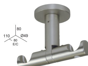
SUPPORT PLAFOND DOUBLE 20-20 mm. (Non disponible en blanc, noir, doré et doré mat)
