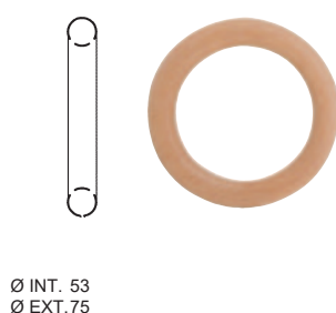
ANNEAU SANS CROCHET
