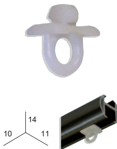
FIXATION INTERMÉDIAIRE
