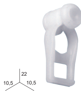
SUSPENDEUR À ROUE
