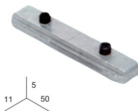
JONCTION METALLIQUE (profilés 950/910)
