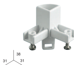
UNION D'ANGLE
