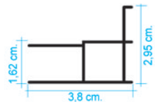
PROFILÉ BARRE TRANSV.
