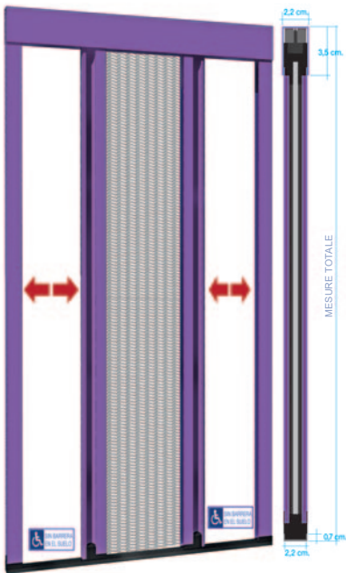
PROFILÉ PORTE RÉVERSIBLE
