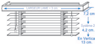
G-3. CANTONNIÈRE EN "U" Installation au mur ou au plafond (STANDARD)
