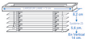
G-4. DOUBLE ENVIRONNEMENT Installation au plafond
