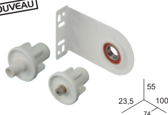
SUPPORT LONG CENTRAL AVEC TRANSMISSION Les 2 stores peuvent se commander avec une seule chaînette
