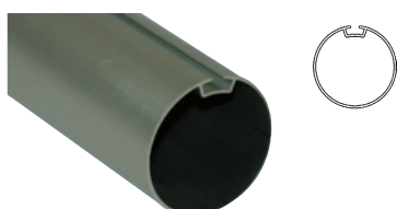
PROFILÉ ALUMINIUM Ø38 (6 m.)
