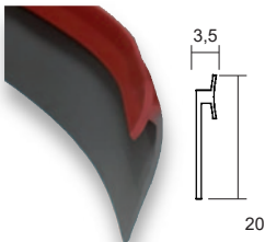
PROFILE PVC DE 6 m.
