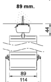
COMMANDE DROITE OUVERTURE à GAUCHE
