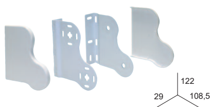
JEU SUPPORT DOUBLE (Gauche)
