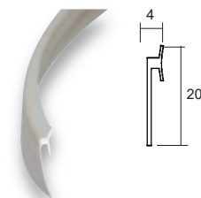
PROFILE PVC DE 6 m.
