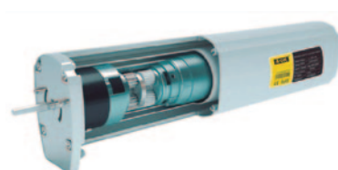
MOTEUR TRINGLE 1,5 N.m POUR BATTERIE EXTERNE
