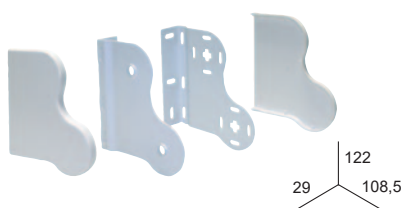
JEU SUPPORT DOUBLE (Droit)
