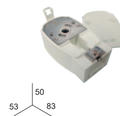
POULIE RETOUR POUR MOTEUR 1,5 N.m
